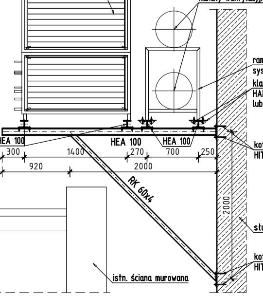
PRZEKRÓJ B-B skala 1:50
