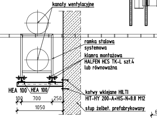
PRZEKRÓJ B-B skala 1:50
